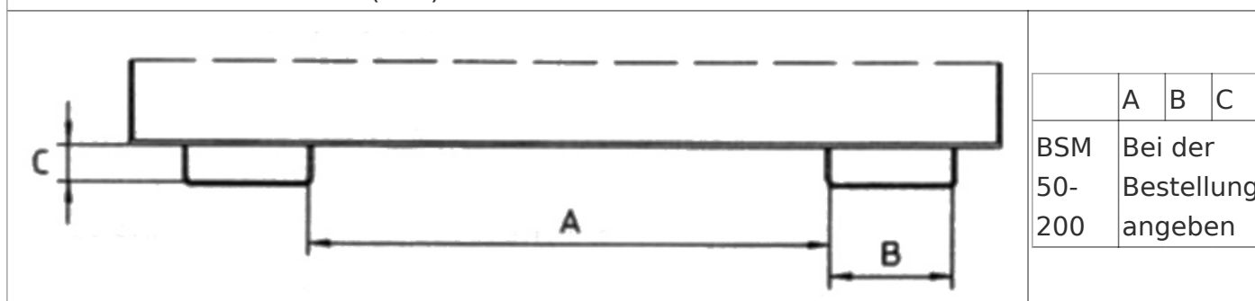
Einfahrtaschen-Innenmaße (mm)
