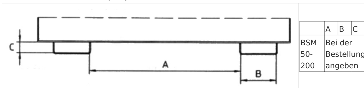
Einfahrtaschen-Innenmaße (mm)
