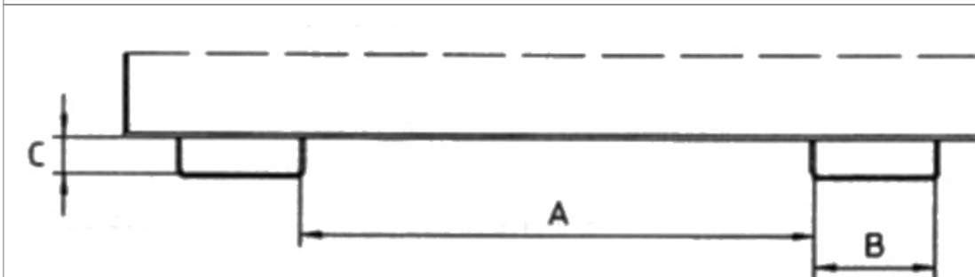
Einfahrtaschen-Innenmaße (mm)
