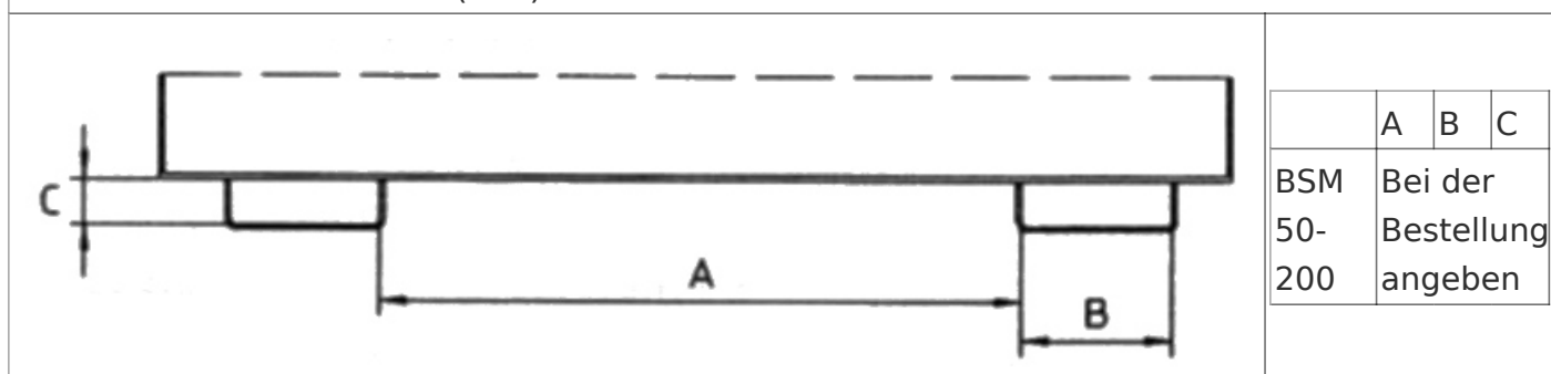
Einfahrtaschen-Innenmaße (mm)
