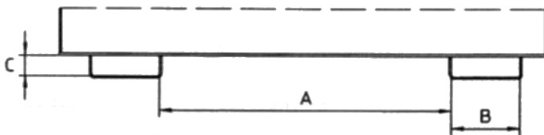
Einfahrtaschen-Innenmaße (mm)
