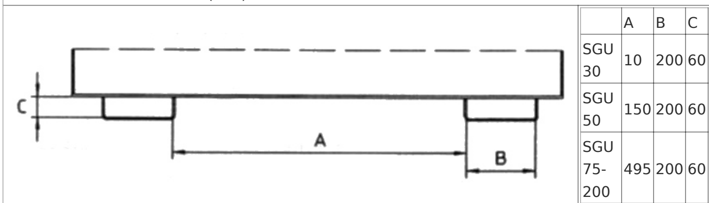
Einfahrtaschen-Innenmaße (mm)
